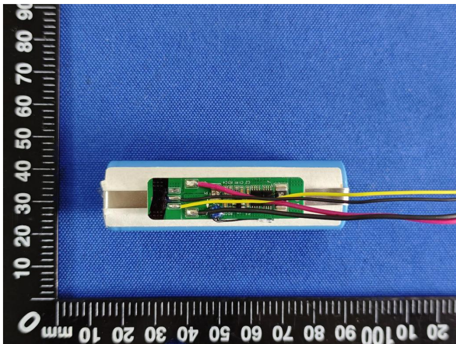
图 3 电池内部
