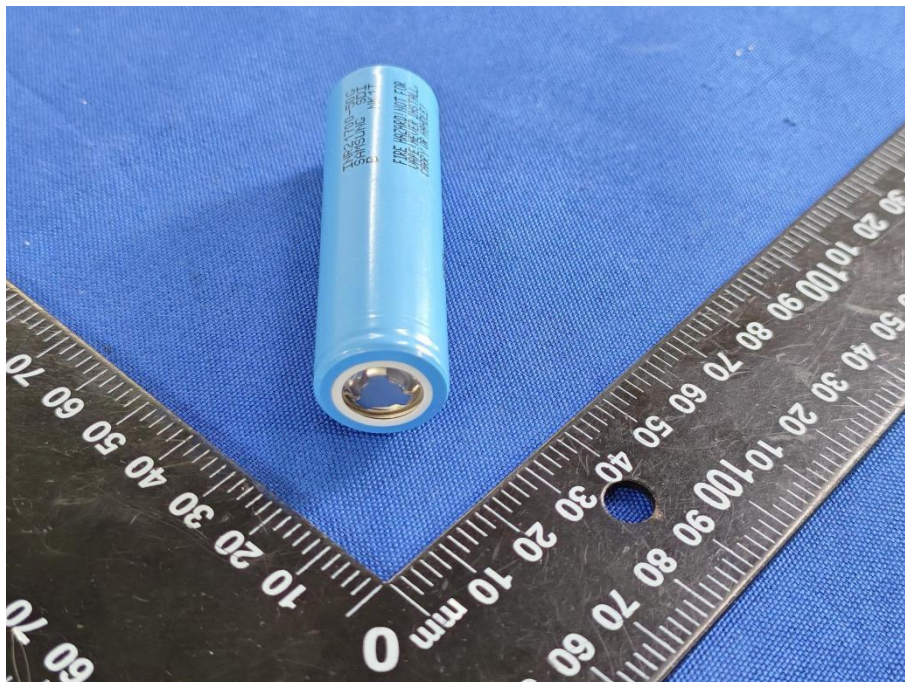
图 7 电芯顶部
