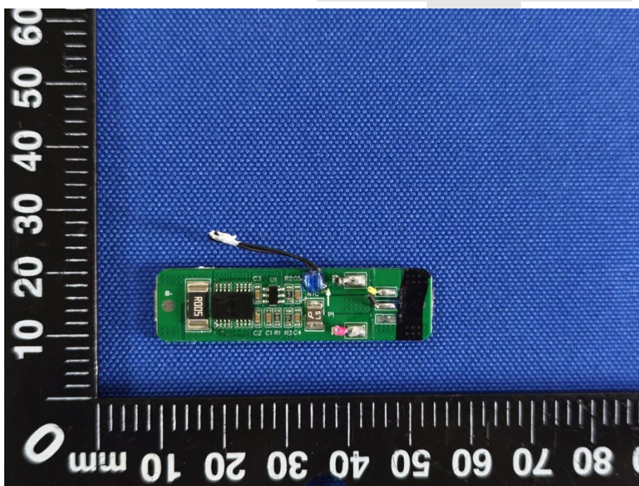
图 4 保护电路正面
