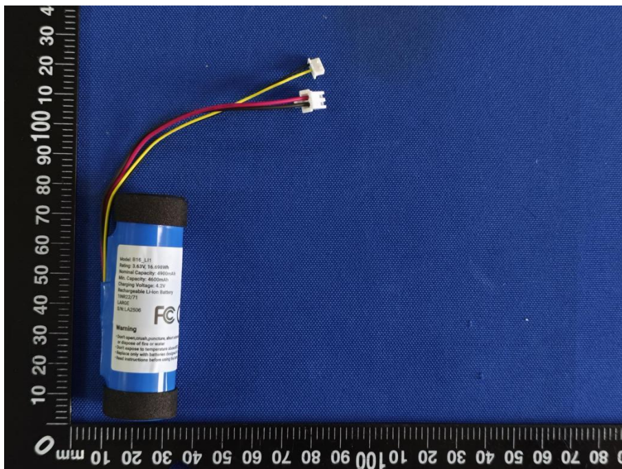
图 1 电池正面
